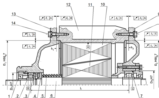
Фиг. 1 Телферен електродвигател с конусен ротор и статор
