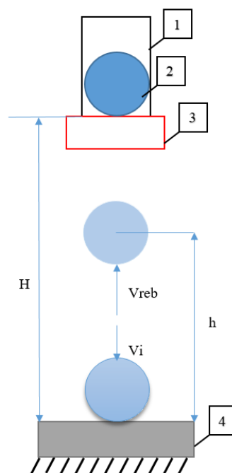
Фиг.1 Схема на опитната постановка
