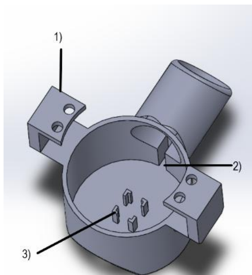
Фиг.6 Разпределително тяло
