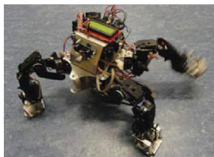
Рис. 7. Робот Winspecbot на базе шагающего магнитного транспортного устройства [8].
